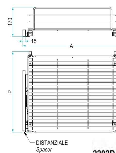
Cassetto estraibile con distanziali - Estrazione manuale. Drawer basket with spacers - Manual extraction.
